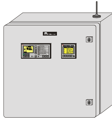
Daljinski terminal DT-10SE za daljinsko vođenje priključka solarne elektrane (do 500kW) na NN postrojenje distribucijske mreže
